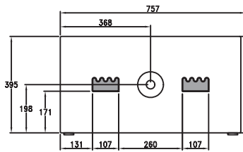
LEFT SIDE
